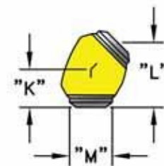
45° Long Sweep Ell (LSE45)
