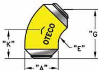
45° Long Sweep Ell (LSE45)
