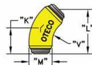
45° Long Sweep Ell (LSE45)
