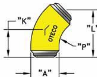
45° Long Sweep Ell (LSE45)
