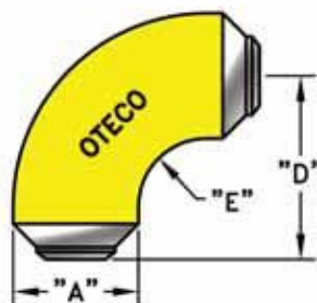
90° Long Sweep Ell (LSE90)
