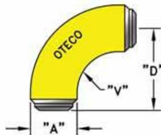
90° Long Sweep Ell (LSE90)
