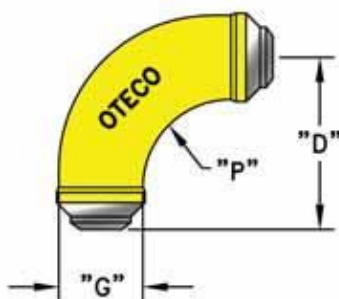
90° Long Sweep Ell (LSE90)
